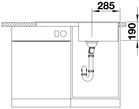
Vooranzicht
