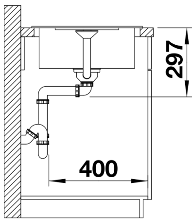
Zijaanzicht
