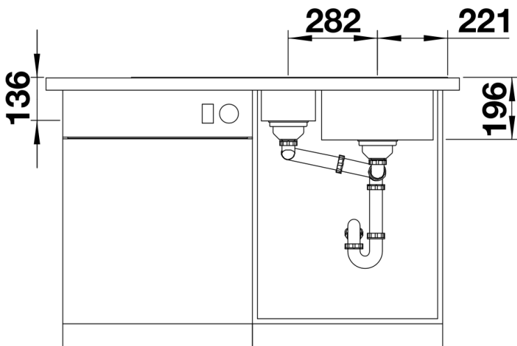
Vooraanzicht
