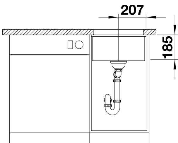
Vooranzicht
