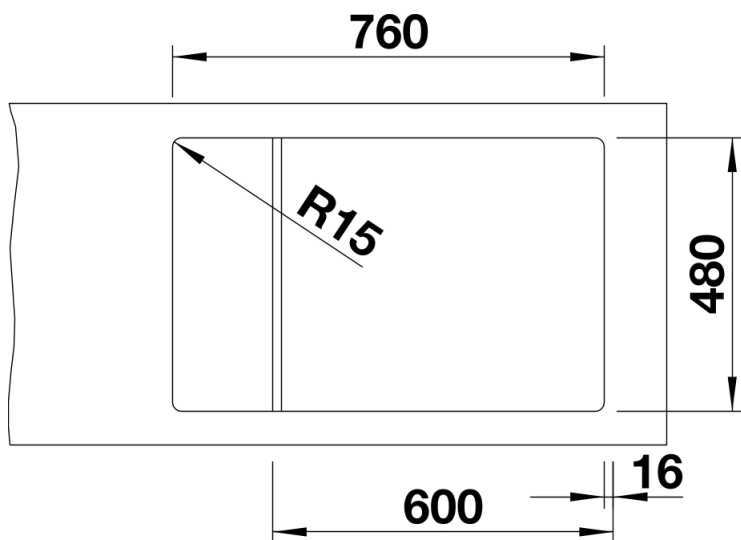
Uitgesneden
