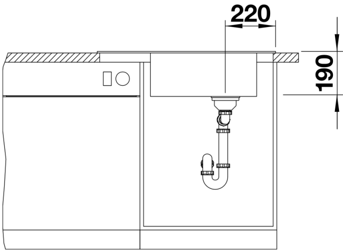
Vooraanzicht
