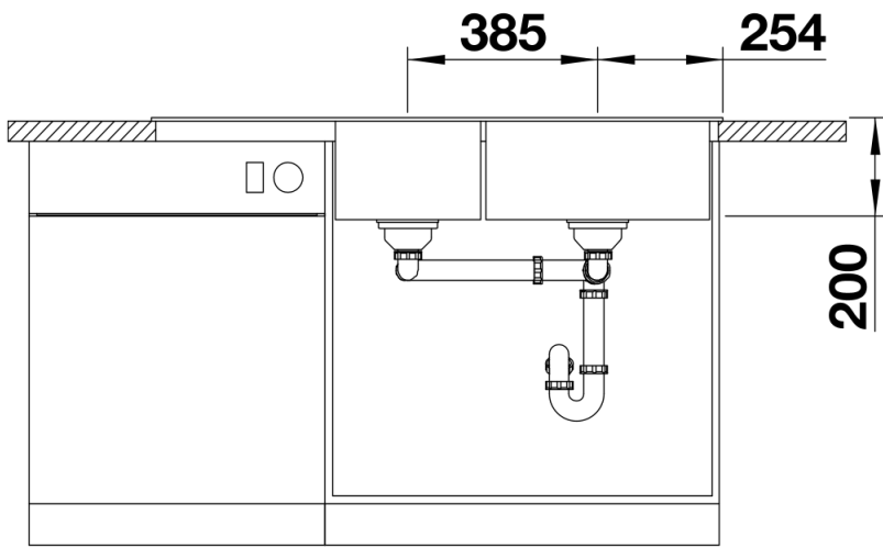
Vooranzicht
