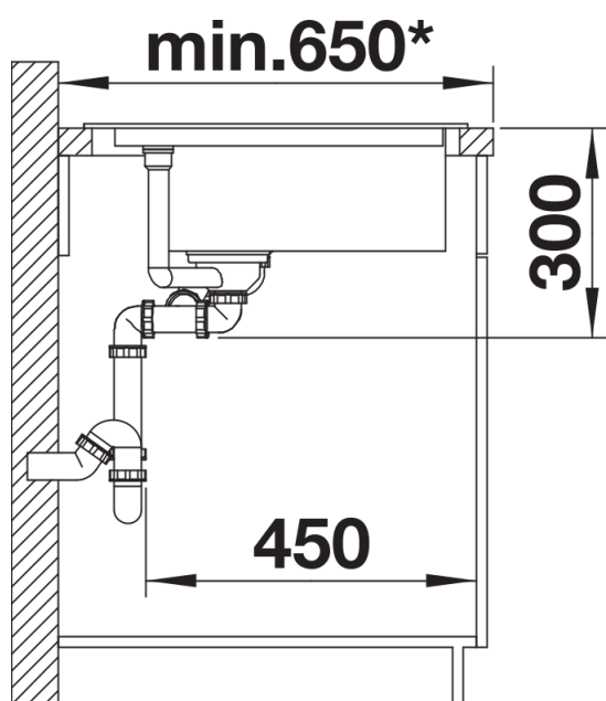
Zijaanzicht
