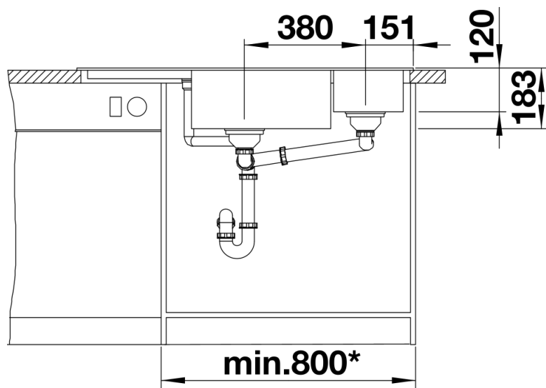
Vooraanzicht
