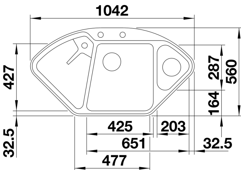
Bovenaanzicht
