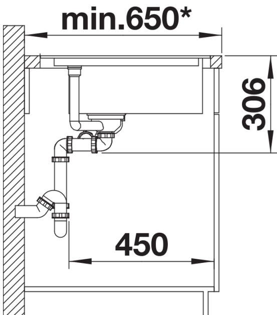
Zijaanzicht
