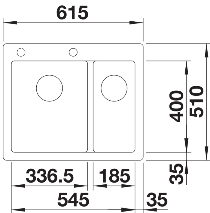
Bovenaanzicht
