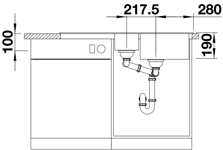
Vooraanzicht
