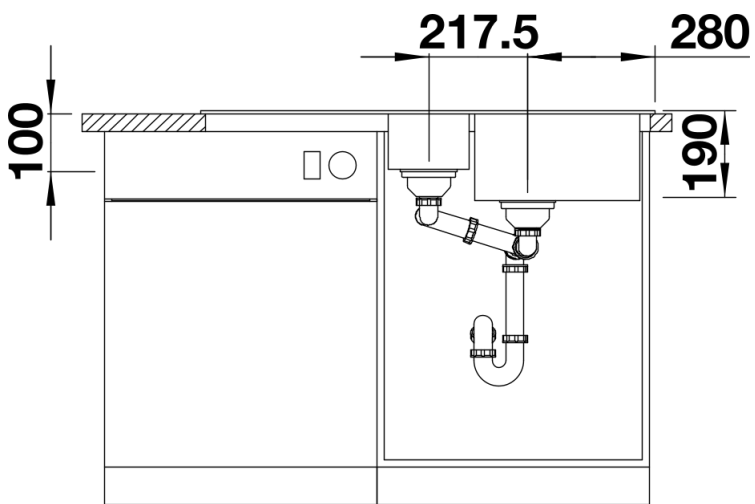
Vooraanzicht
