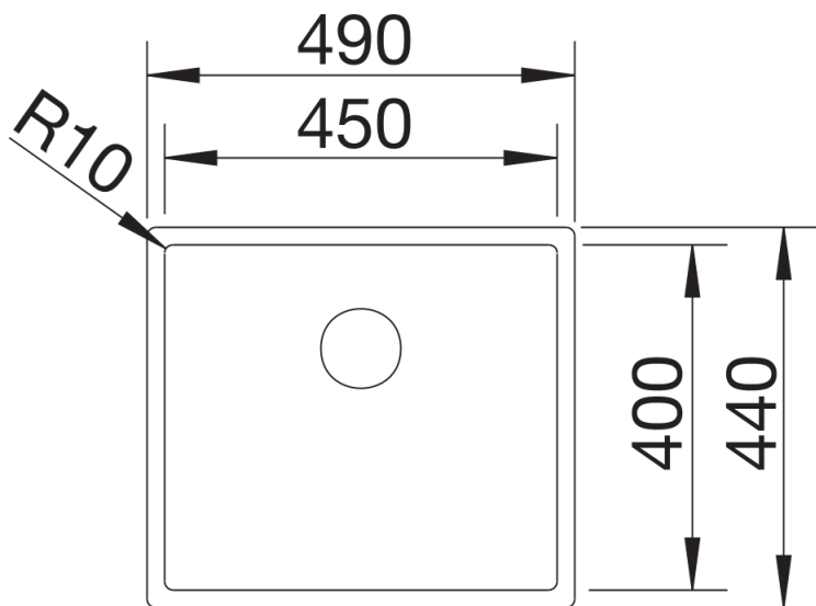
Bovenaanzicht
