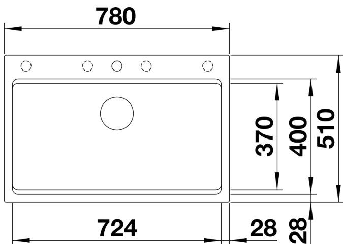
Bovenaanzicht
