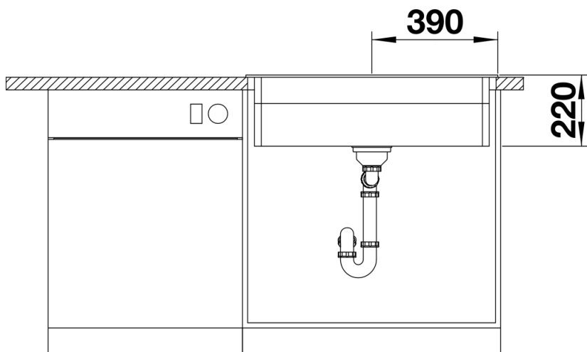
Vooranzicht
