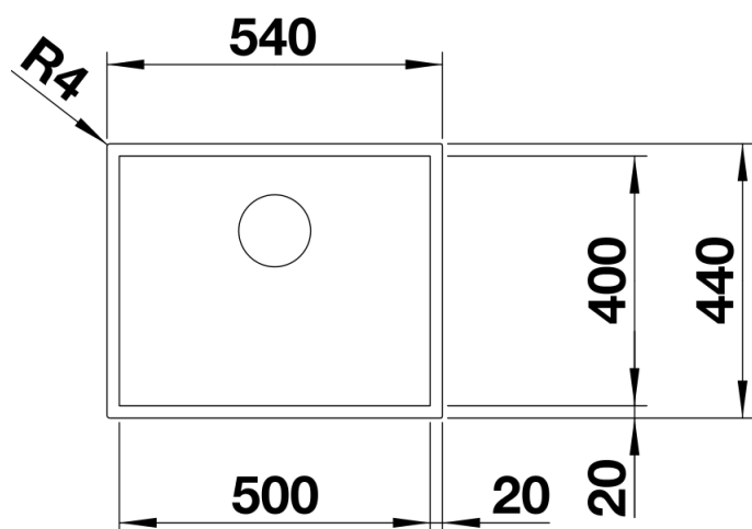
Bovenaanzicht
