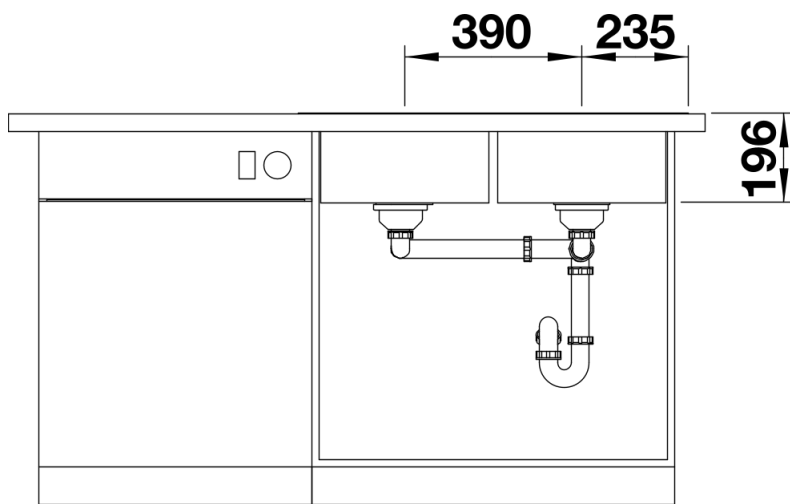
Vooranzicht
