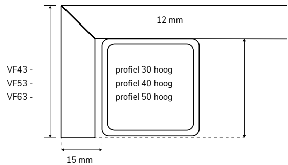
Afbeelding blad over frame (liggers frame niet zichtbaar)
