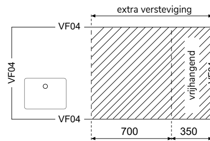
Voorbeeld situatie B perspectief en bovenaanzicht werkblad.
