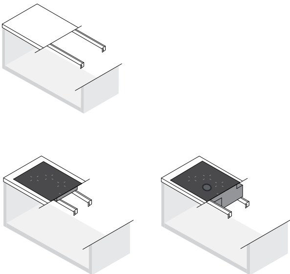
Voorbeeld ondersteuningsset (DIV-STEUN-GR) ter ondersteuning van kookplaat >20 KG
