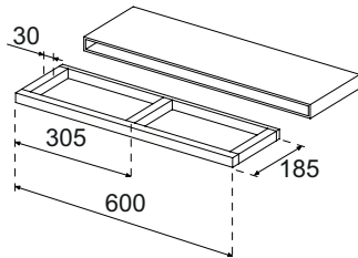
Technische tekening bevestigingsframe wandplank 600 mm (artikel 180129)
