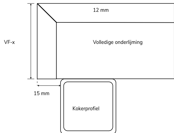
Afbeelding blad op frame (liggers frame zichtbaar)
