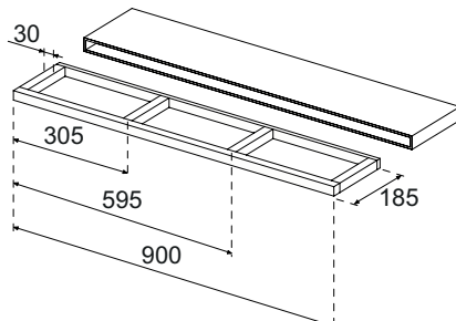
Technische tekening bevestigingsframe wandplank 900 mm (artikel 180130)
