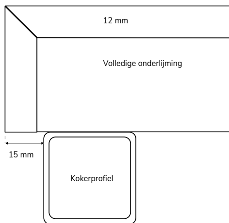
Afbeelding blad op frame (liggers frame zichtbaar)
