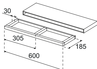
Dessin technique du cadre de fixation de l'étagère murale 600 mm (article 180129)
