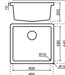
Encastré/sous-encastré
