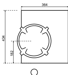
Dessus Côté
