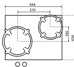
Dessus Côté
