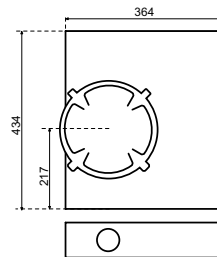
Face avant
