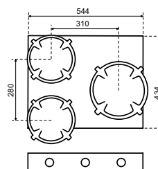
Face avant
