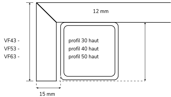
Illustration du plan de travail sur la structure (les poutres du cadre ne sont pas visibles)
