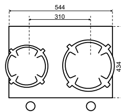
Dessus Côté
