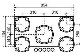
Dessus Côté
