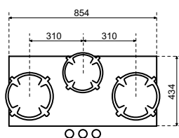
Dessus Côté
