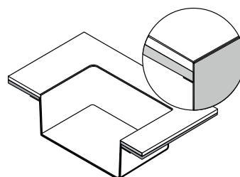
Rimless (RIM)
