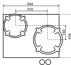
Dessus Côté
