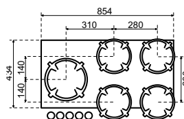
Dessus Côté
