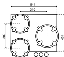
Dessus Côté
