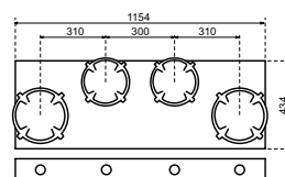
Face avant
