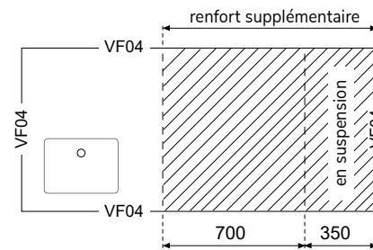
Exemple de situation B : perspective et vue de dessus du plan de travail.
