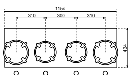
Dessus Côté
