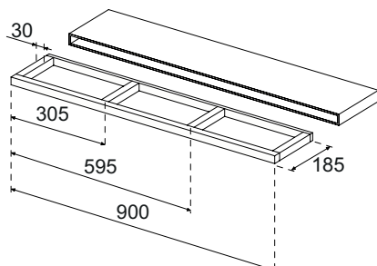
Dessin technique pour la fixation de l'étagère murale 900 mm (article 180130)
