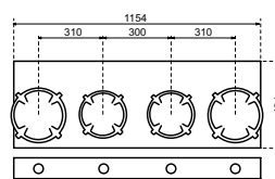
Face avant
