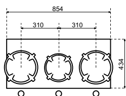
Dessus Côté
