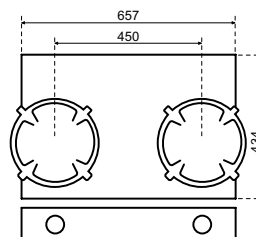
Face avant
