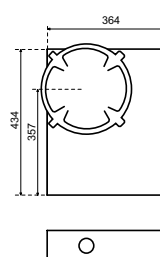
Face avant
