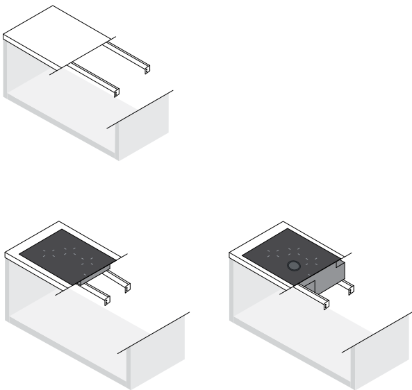
Exemple de kit de support (DIV-STEUN-GR) pour supporter une table de cuisson >20 KG
