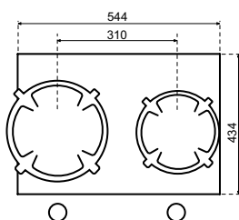
Dessus Côté
