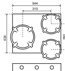
Face avant
