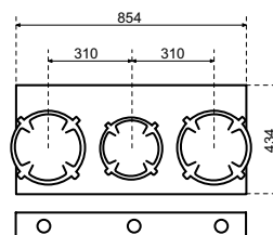
Face avant
