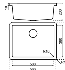
Encastré/sous-encasté
