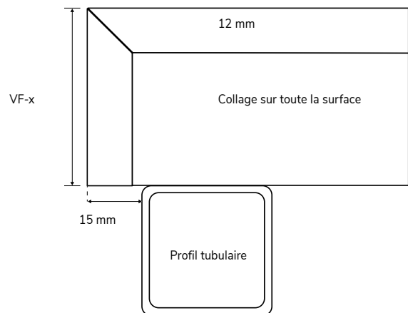
Illustration du plan de travail sur la structure (les poutres du cadre ne sont pas visibles)
