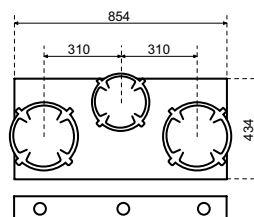
Face avant
