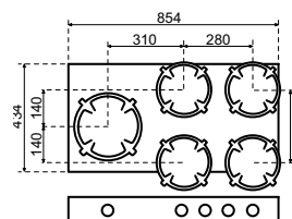
Face avant
