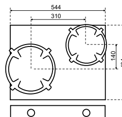
Face avant
