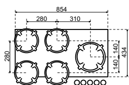
Dessus Côté
