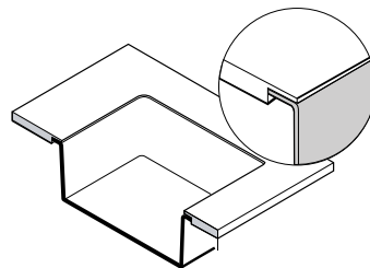
Semi-onderbouw (SON)
